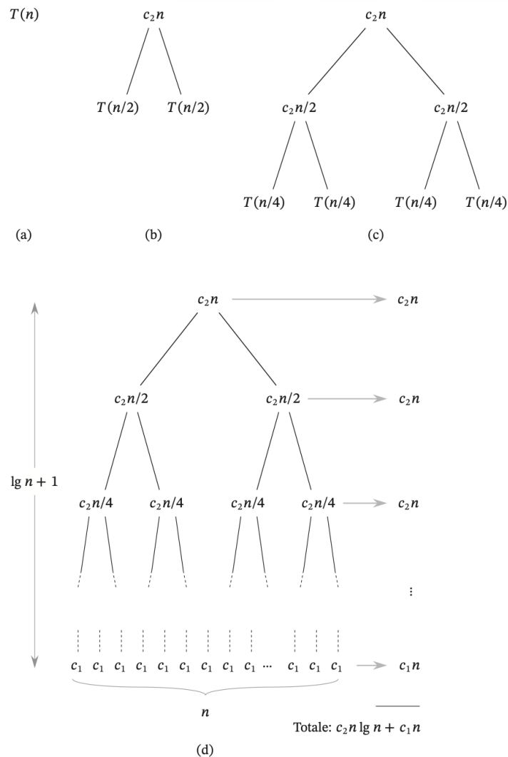
La costruzione di un albero di ricorsione per la ricorrenza T(n) = 2T(n/2) + cn . La parte (a) mostra T(n) , che viene progressivamente espanso in (b)-(d) per formare l'albero di ricorsione. L'albero completamente espanso nella parte (d) ha \lg n + 1 livelli. Ogni livello al di sopra di quello delle foglie contribuisce per un costo complessivo di c_2n , mentre il livello delle foglie ha un contributo di c_1n . Di conseguenza, il costo totale è c_2n \lg n + c_1n = \Theta(n \lg n) .
